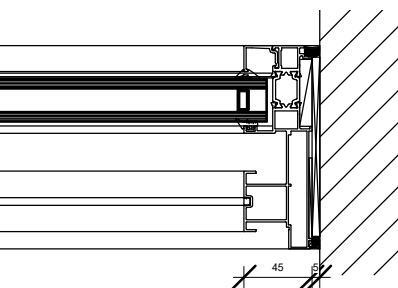
5 Detail 3 1 : 5
