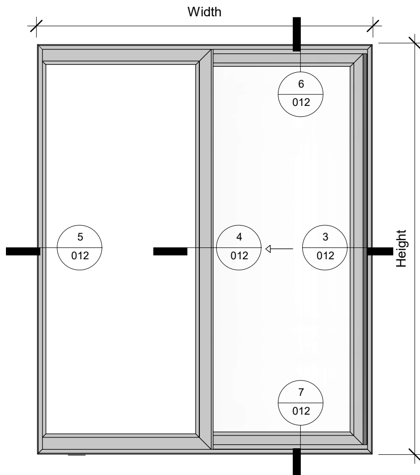
2 Elevation Back 1 : 20
