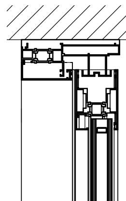
6 Detail 4 1 : 5
