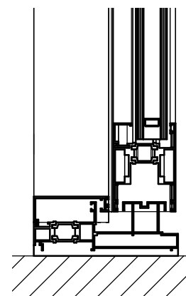
7 Detail 5 1 : 5
