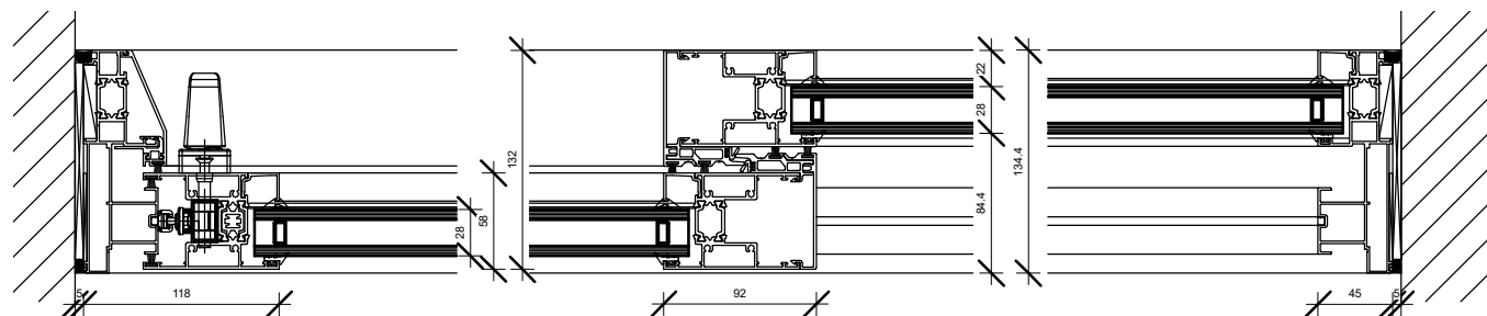
3 Detail 1 1 : 5
