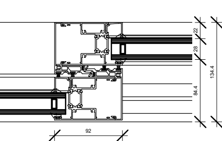
4 Detail 2 1 : 5
